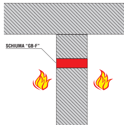
PARETE / PARETE
