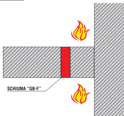
SOLAIO / PARETE
