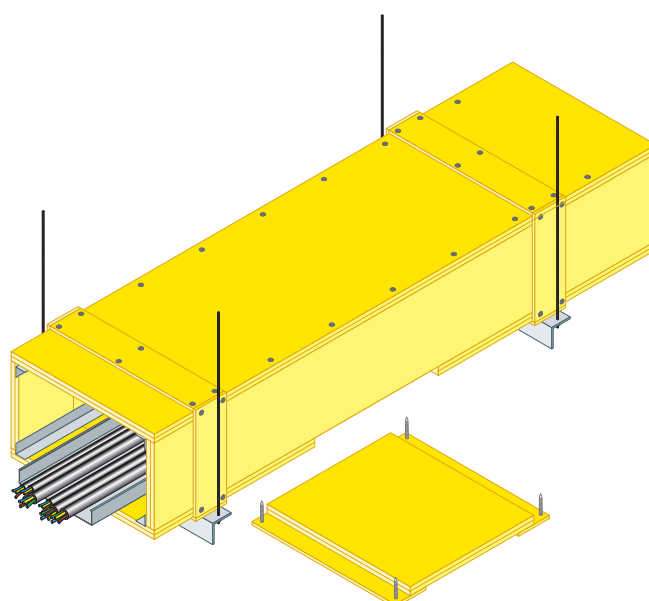
PANNELLO DI ISPEZIONE INFERIORE
