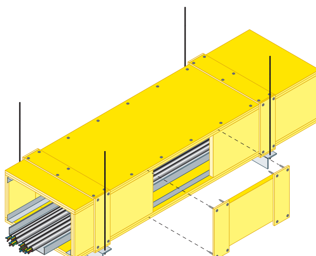
PANNELLO DI ISPEZIONE LATERALE
